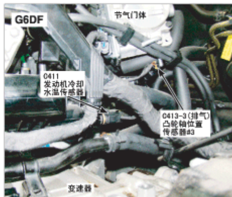
183. 发动机左侧
