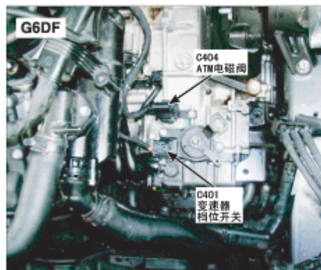
184. 变速器
