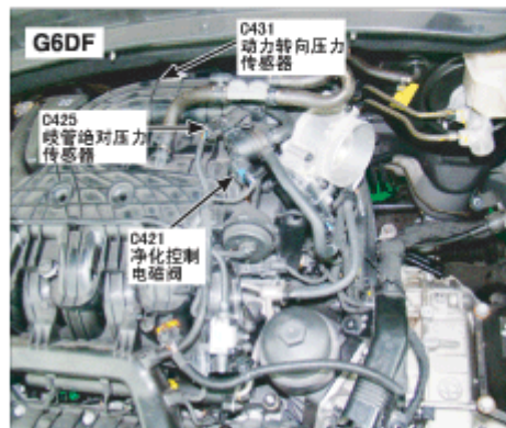
181. 发动机顶部
