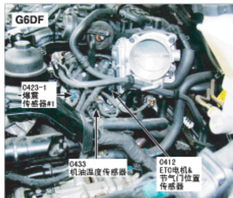
182. 发动机左侧
