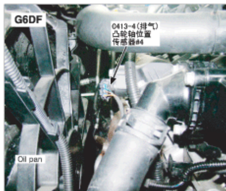
186. 发动机前部
